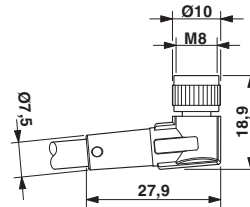
Dessin coté
