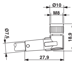
Dessin coté
