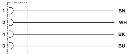
Affectation des contacts du connecteur femelle M8
