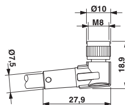
Dessin coté
