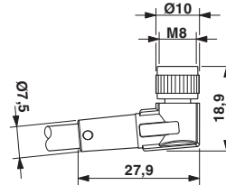
Dessin coté
