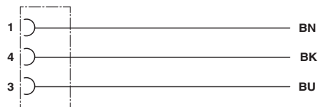
Schéma de connexion
