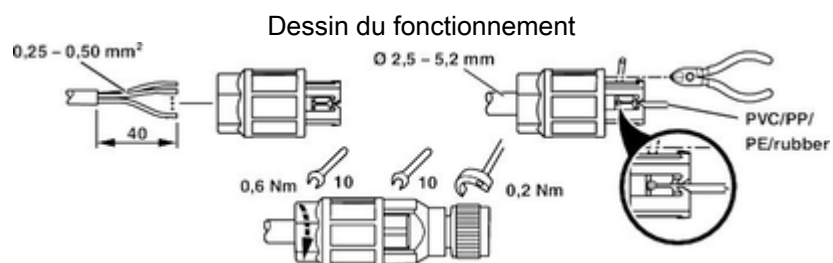
Dessin schématique
