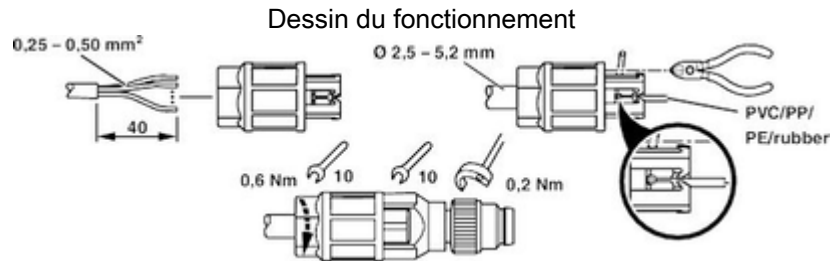
Dessin schématique
